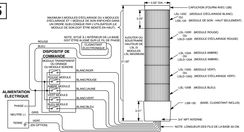
SCÉNARIO D'INSTALLATION MONTRANT LES MODULES D'ÉCLAIRAGE ROUGE ET VERT CÂBLÉS À UN CLIGNOTANT. LES AUTRES MODULES D'ÉCLAIRAGE SONT FIXES LORSQU'ALLUMÉS. LE CLIGNOTANT EST POUR UTILISATION UNIQUEMENT AVEC MODULES D'ÉCLAIRAGE 120V CA. LE MODULE DE SON NE PEUT ÊTRE CÂBLÉ AU CLIGNOTANT. 29043371E
