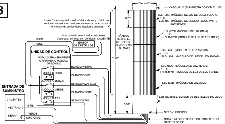
MUESTRA DE INSTALACION DE LOS MÓDULOS DE LUZ ROJO Y VERDE CONECTADOS AL EMISOR DE DESTELLOS. LOS OTROS MÓDULOS FUNCIONAN A NIVEL MEDIO CUANDO SE ENCIENDEN. EL EMISOR DE LUZ DEBE UTILIZARSE SÓLO CON MÓDULOS DE LUZ DE 120VAC. NO SE PUEDE CONECTAR EL MÓDULO DE SONIDO AL EMISOR DE DESTELLOS. 29043273E
