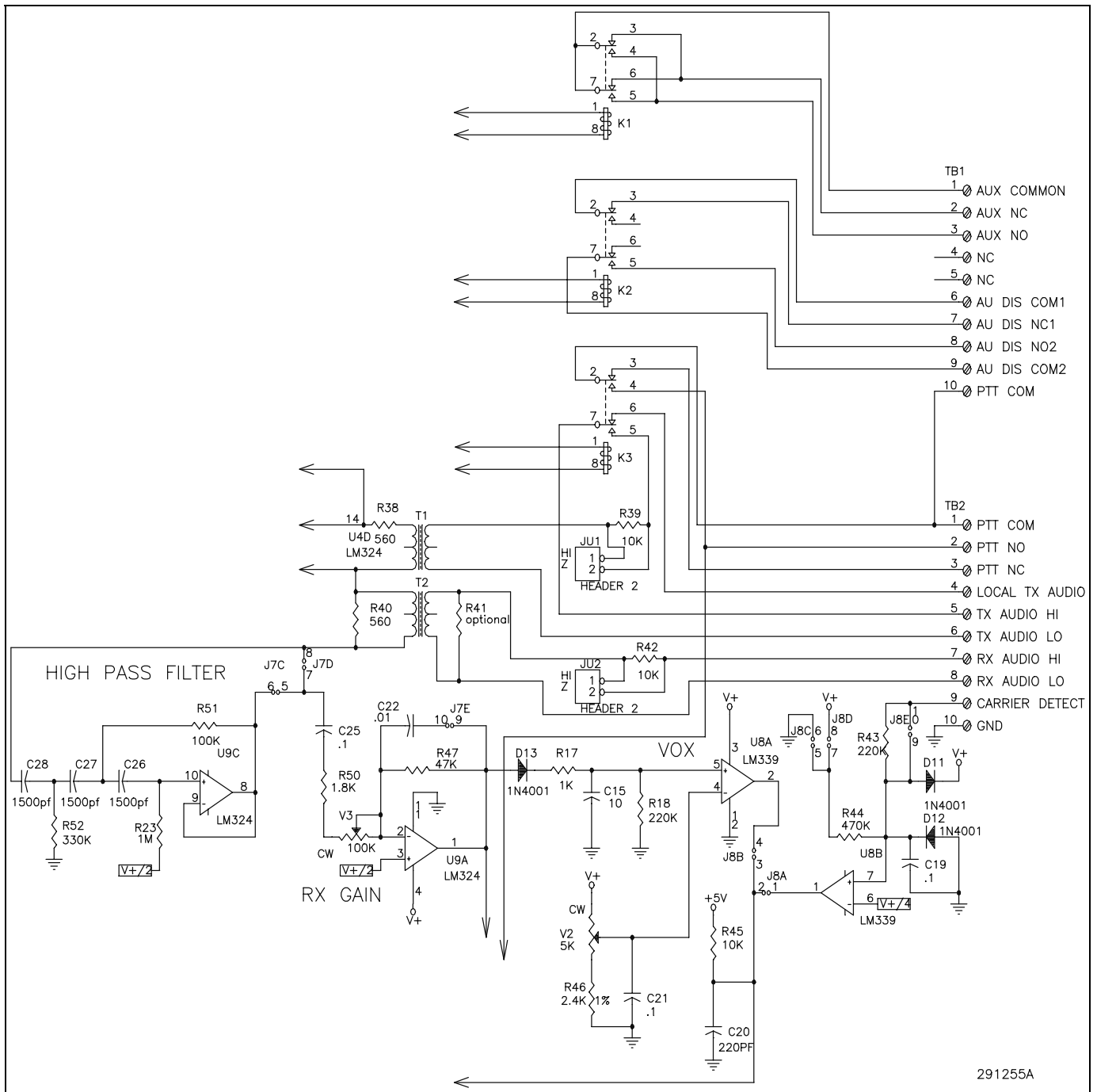
Fig. 4.2: I/O Schematic
